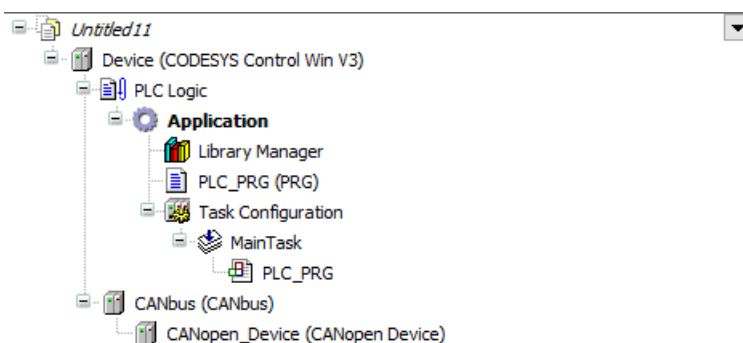
Bild 1: Gerätebaum
